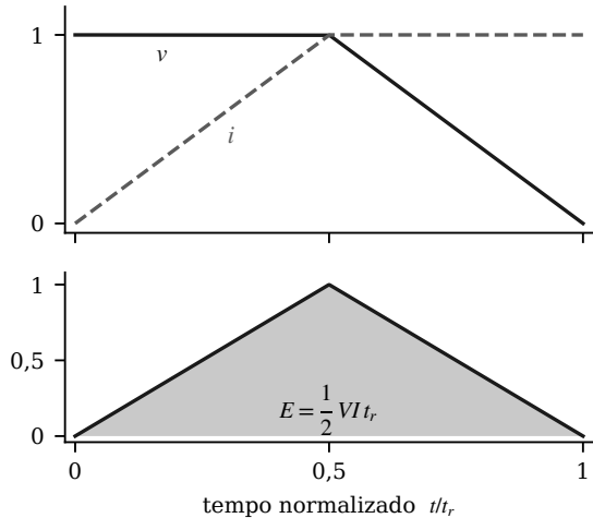
(b) carga indutiva grampeada
